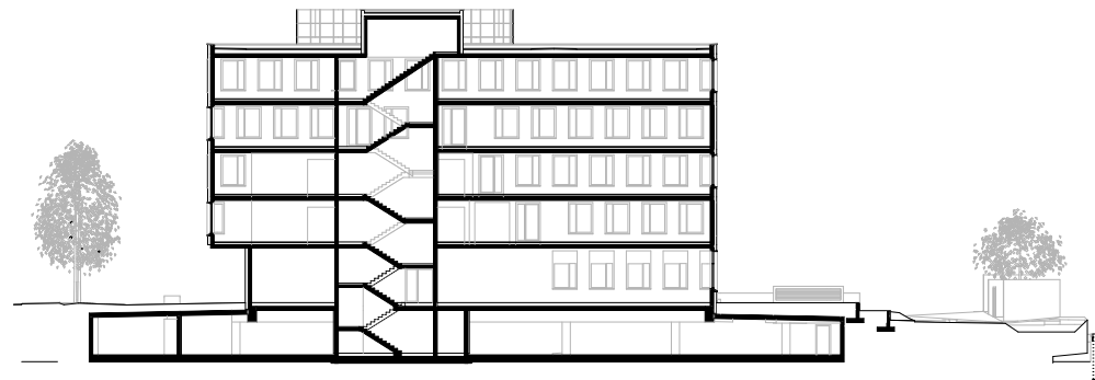
BF1 Regelschnitt
